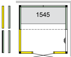
Panacea 1717 dim. : 1700 x 1700 mm
