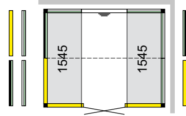
Panacea 2117-2B dim. : 2100 x 1700 mm
