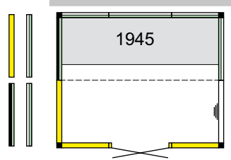
Panacea 2117-1B dim. : 2100 x 1700 mm
