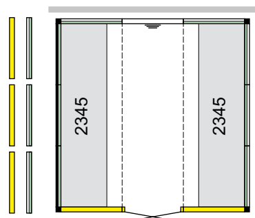
Panacea 2525-2B dim. : 2500 x 2500 mm
