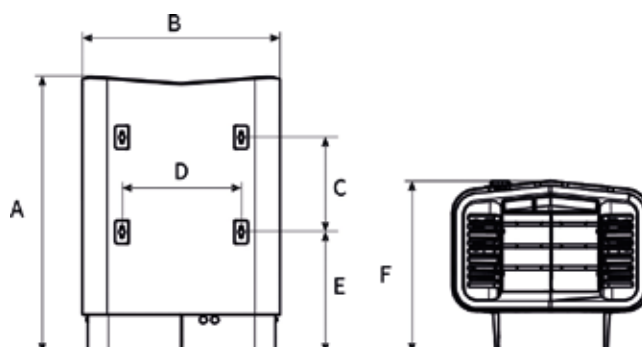
Dimensions des poêles (cf tableau ci-dessus)
